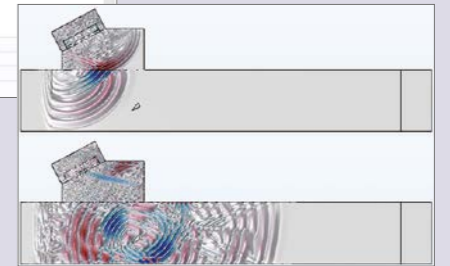
不連続ガラキン法 (DG) による陽的時間発展の NDT (非破壊検査)
